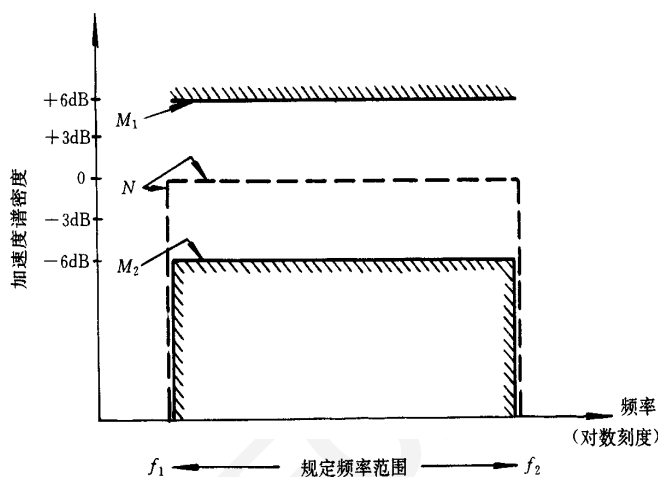
图 4 加速度谱密度的频谱和容差范围
